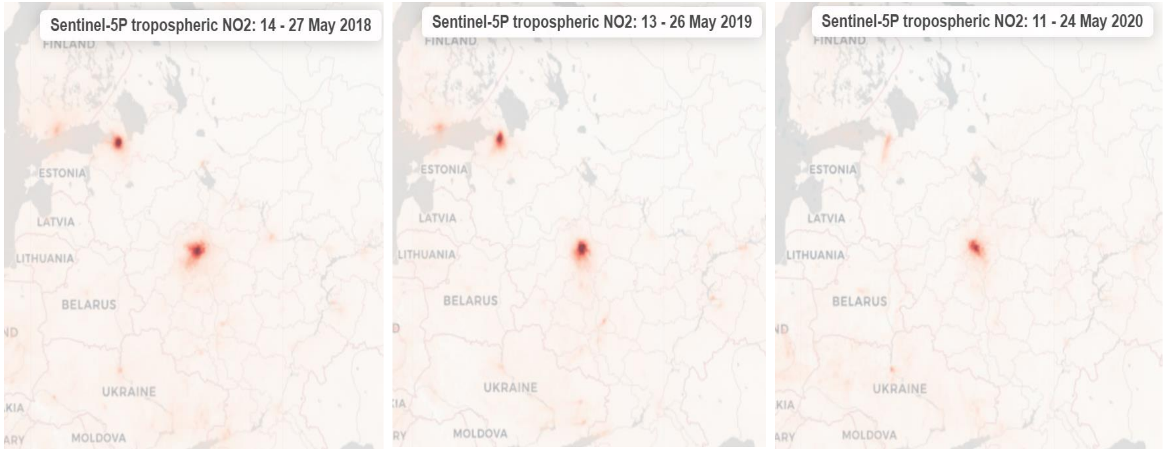
Figuur 1 Driemaal dezelfde uitsnede van Europa waarin je de gemiddelde NO 2 -meting ziet van 14 dagen over een vergelijkbare periode in mei 2018, 2019 en 2020.
