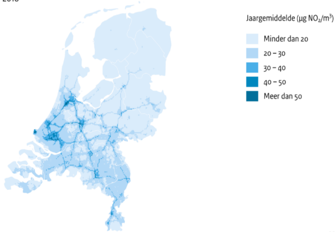
Figuur 1. De gemiddelde gemeten concentratie van stikstofoxiden ( \text{NO}_x uitgedrukt als stikstofdioxide, \text{NO}_2 ) door regionale stations in 2018. Bron: Compendium voor de leefomgeving ( https://www.clo.nl/indicatoren/nl0493-stikstofoxiden )
